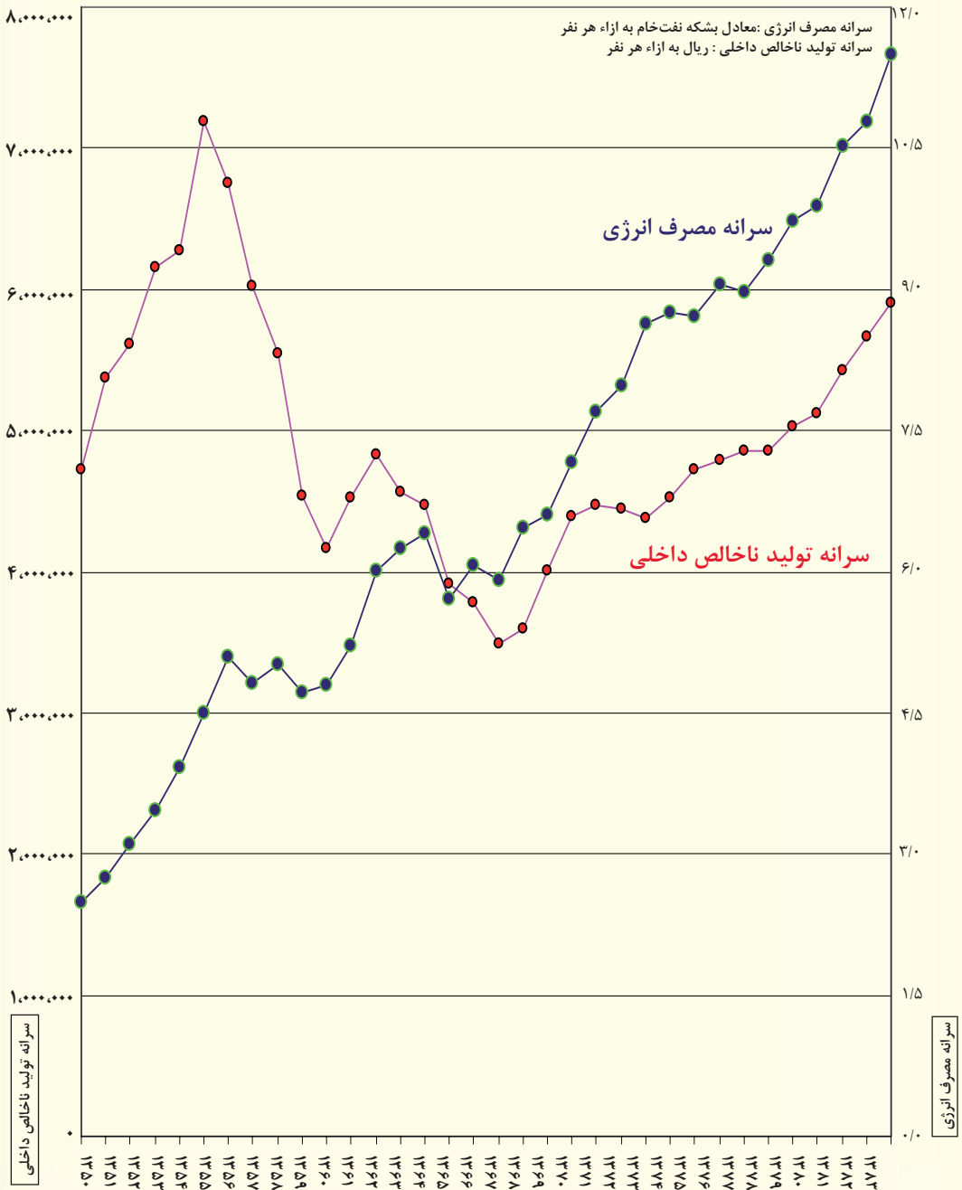
نمودار مقایسه سرانه تولید ناخالص داخلی با سرانه مصرف انرژی طی سال‌های ۱۳۵۰-۱۳۸۳
