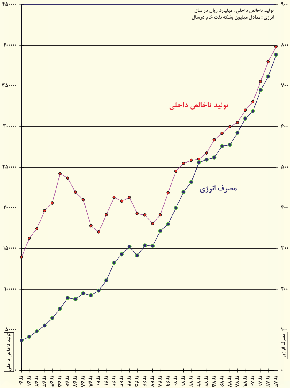
نمودار مقایسه تولید ناخالص داخلی با مصرف انرژی طی سال‌های ۱۳۵۰-۱۳۸۳
