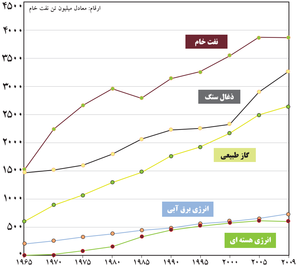
نمودار مقایسه مصرف انرژی‌های اولیه در جهان طی سال‌های ۱۹۶۵-۲۰۰۹
